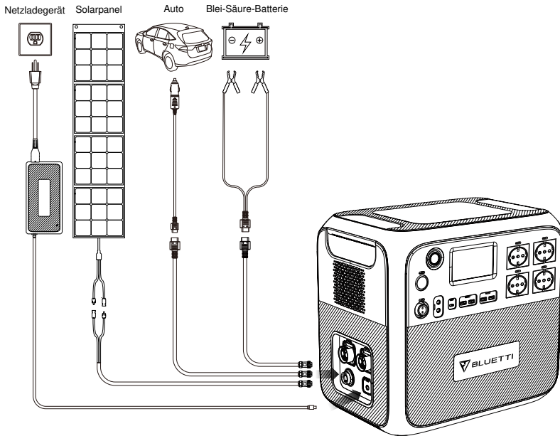
AC200MAX- Doppellaufladungssystem
