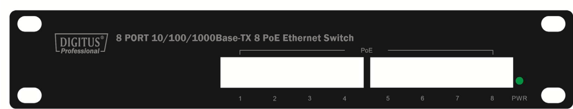
Abbildung 1. Ansicht der Frontblende
